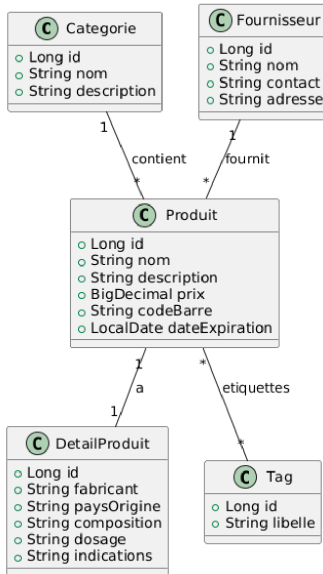
Figure 1 : diagramme de classe
